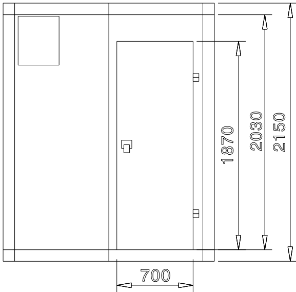
Zij aanzicht
